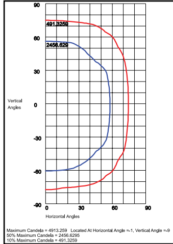
AL35QF1X126UHAC 120°H x 120°V, NEMA 7H x 7V
