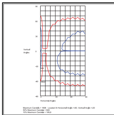
EP10H70R120L
