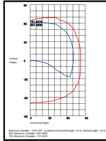
KH25QC1X36UHAC 120°H x 70°V Beam, NEMA 7H x 7V
